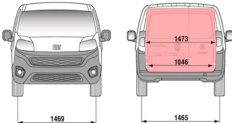
Габаритні розміри та розміри вантажного відділення, мм
